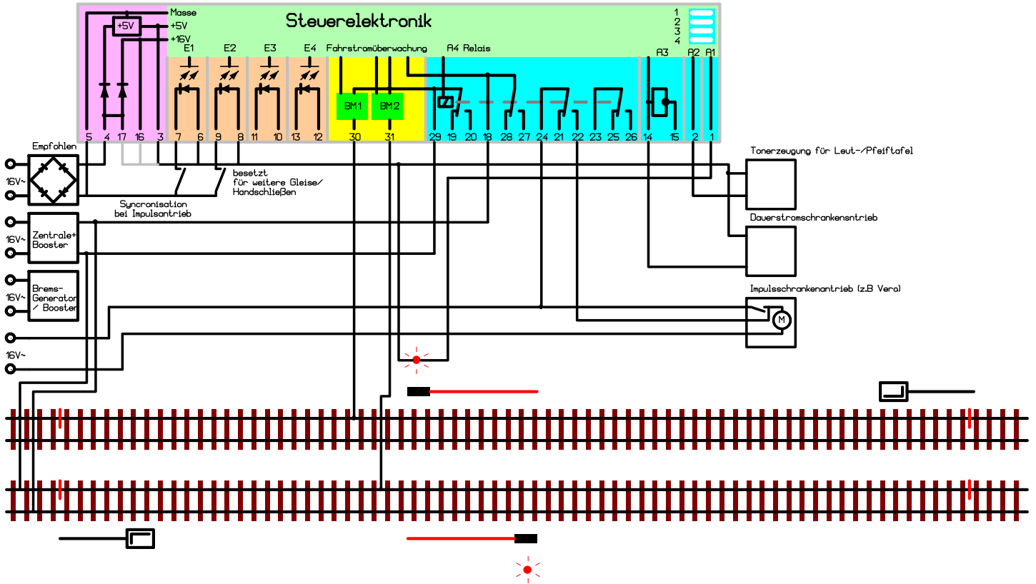
Schrankensteuerung
